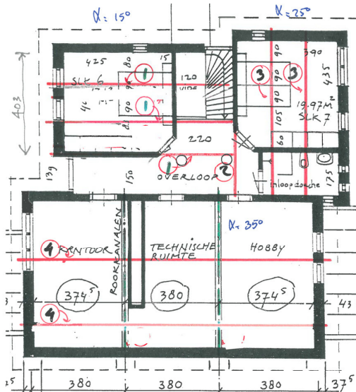
Dakconstructie
