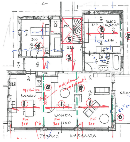
verdiepingsvloer
