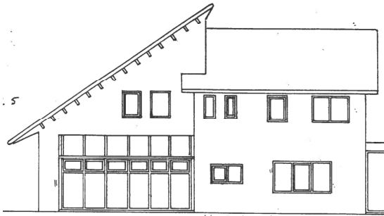
Oostgevel
